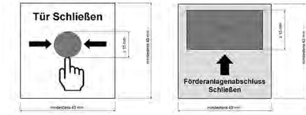
Bild 1: Beispiele für die Gestaltung von Handauslösetastern als Folientaster
